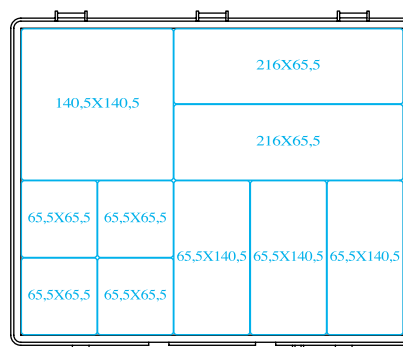
CLASS 42 con 10 vaschette estraibili
