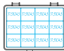
CLASS 19 Con 12 vaschette estraibili
