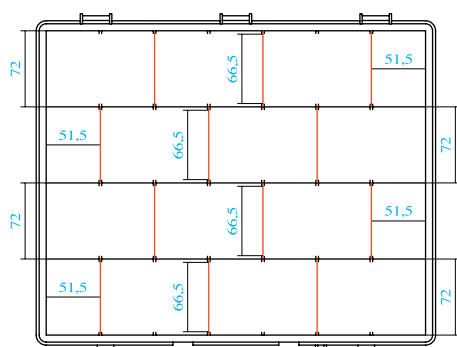
CLASS 41 con 12 divisori estraibili
