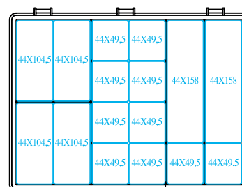
CLASS 32 con 16 vaschette estraibili
